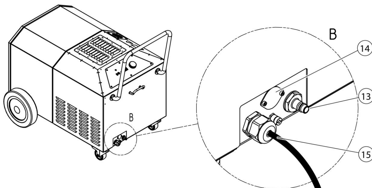
Рис. 2: Подключения
