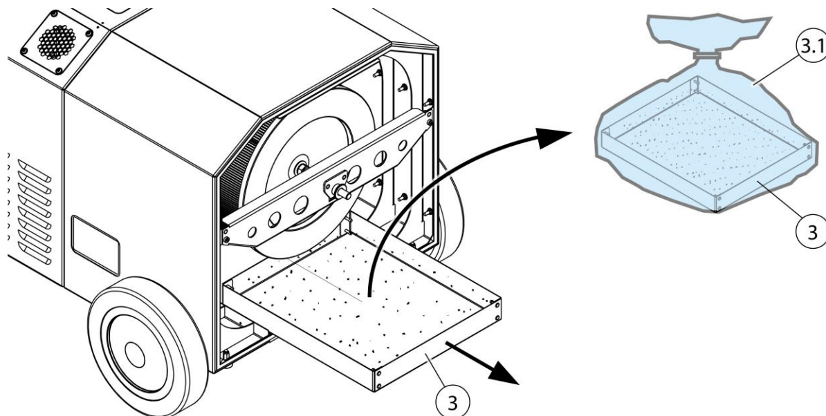
Рис. 7: Замена пылесборника
