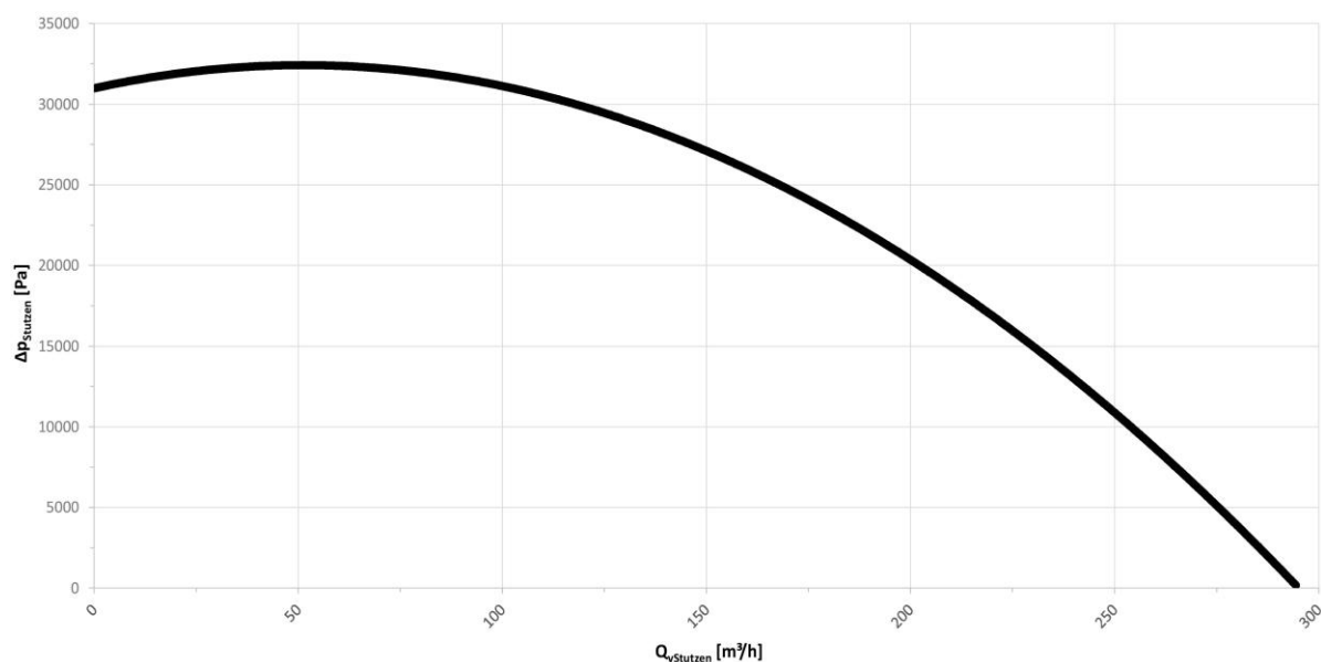
Рис. 16: Характеристика
